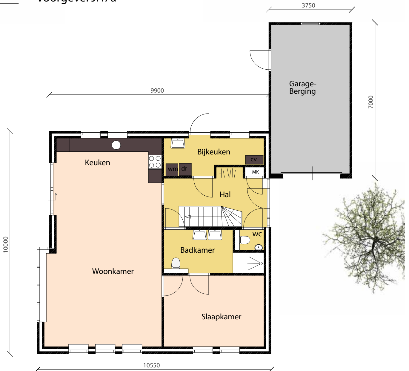
Begane grond
