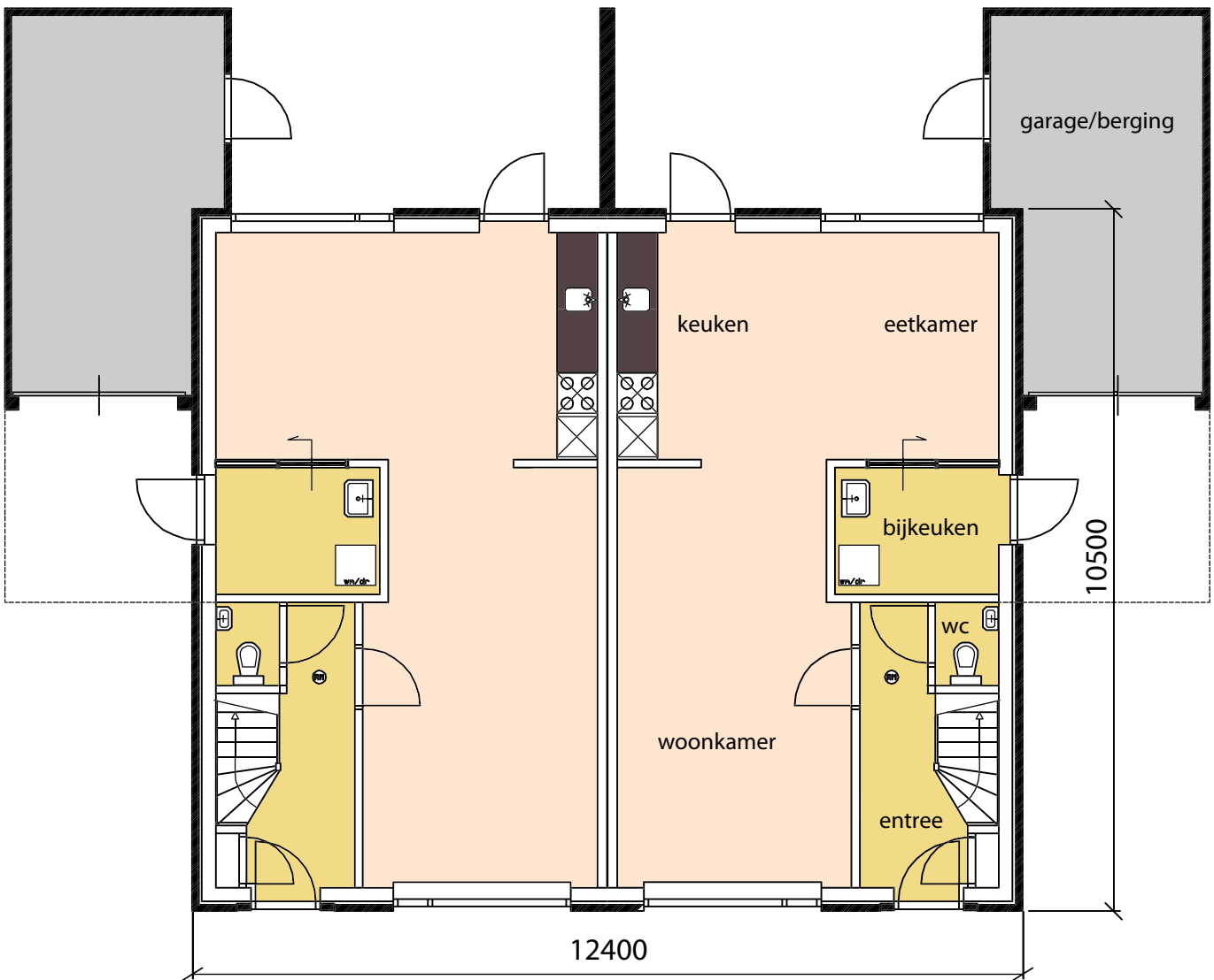
Begane grond
