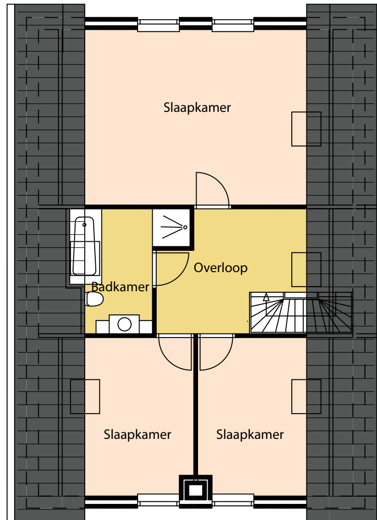
Verdieping
